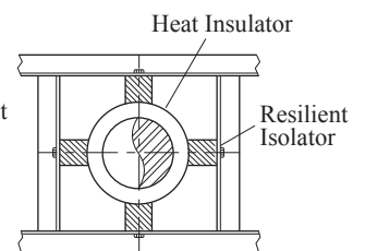
Sway brace ( -+- )
