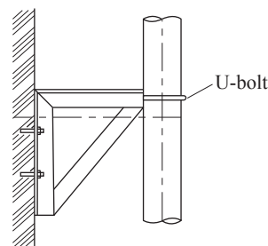
Sway brace ( -+- )
